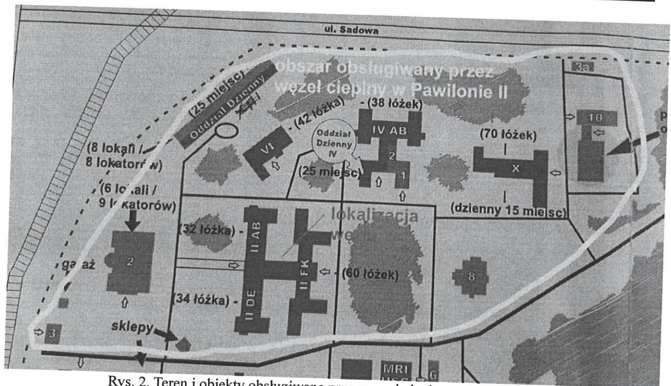
Rys. 2. Teren i obiekty obsługiwane przez węzeł ciepły w Pawilonie II
